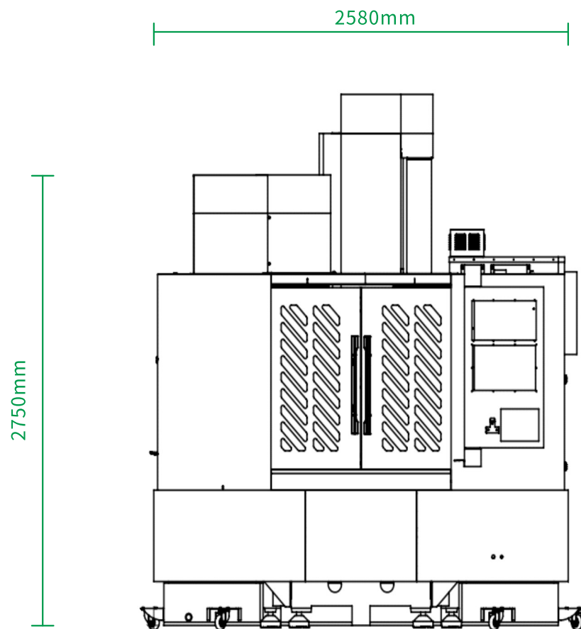
前视图
