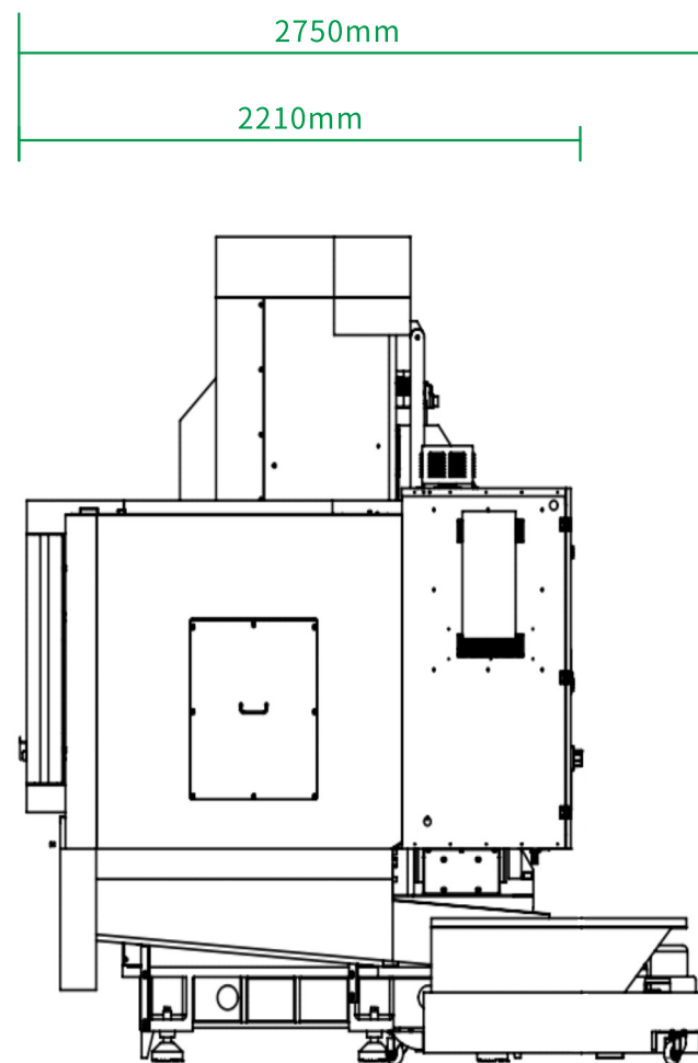
侧视图
