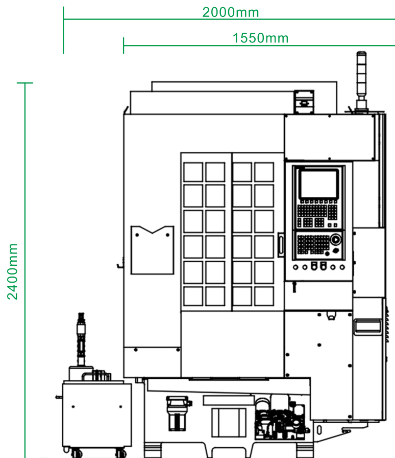
前视图
