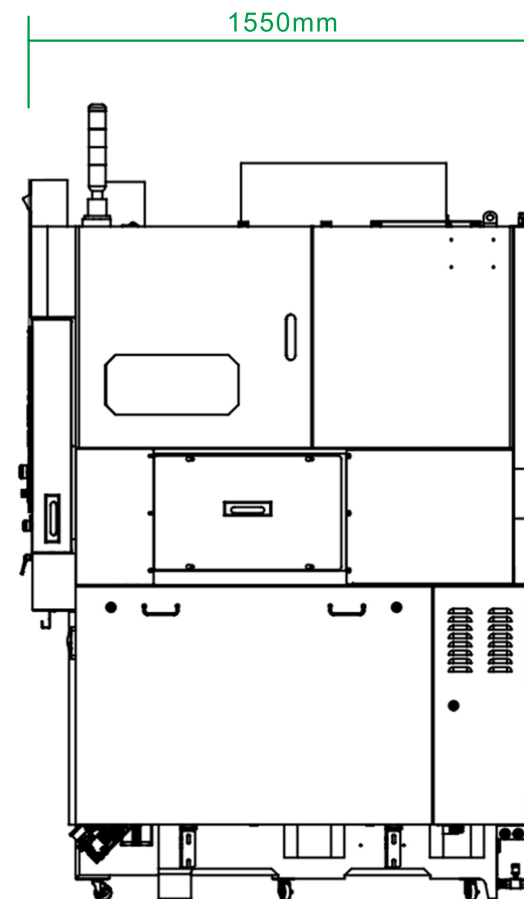
侧视图
